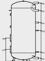
AL 750/R2_C
