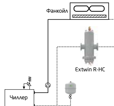
Extwin R-NC - пример монтажа
