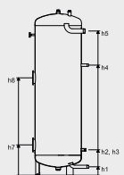
AL 300/R2_C
