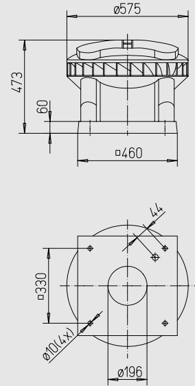
Размеры в мм
