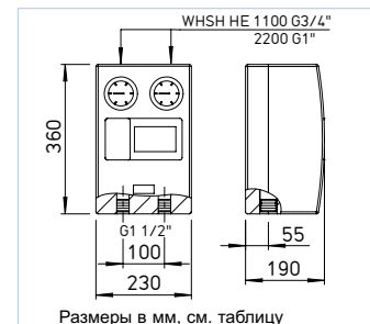
Размеры в мм, см. таблицу
