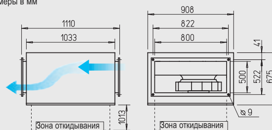
Зона откидывания
