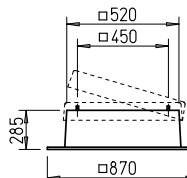
Цоколь для плоской крыши, откидной FDS 250
