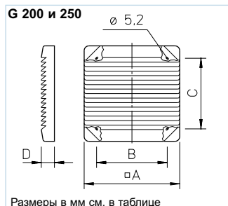
Размеры в мм см. в таблице
