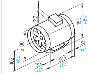
Размеры в мм В 100 В, *MV 100 A
