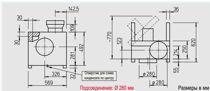
Подсоединение: Ø 280 мм Размеры в мм
