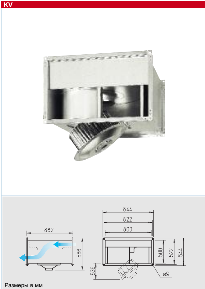
Размеры в мм
