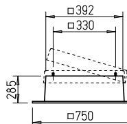
Цоколь для плоской крыши, откидной FDS 225
