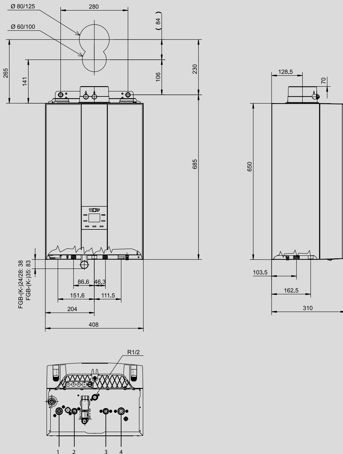
Рис. 1.1 Размеры FGB-(K-)
