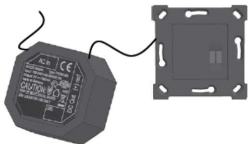
Блок питания для скрытого монтажа с настенным крепежом (Арт. №: 1150692)
